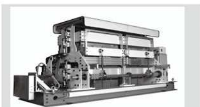
サーボモータ付電子ジャカード
